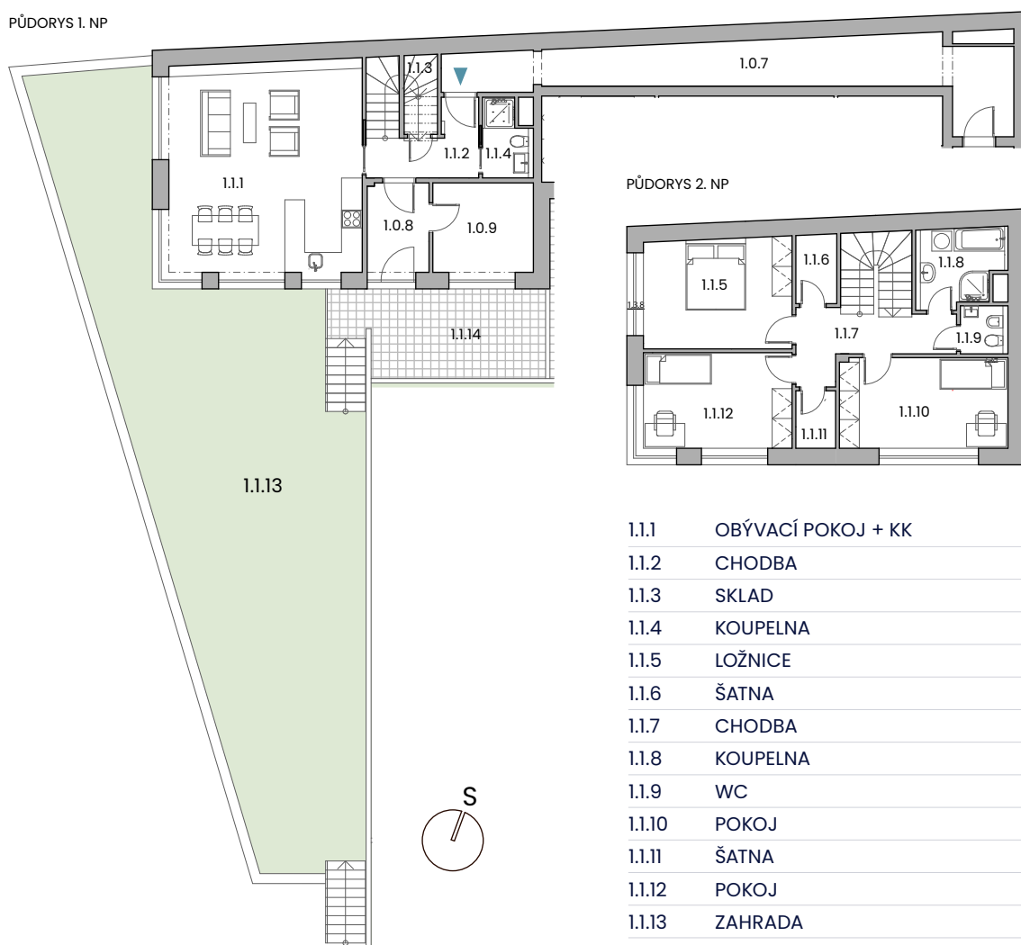
PŮDORYS 1. NP
